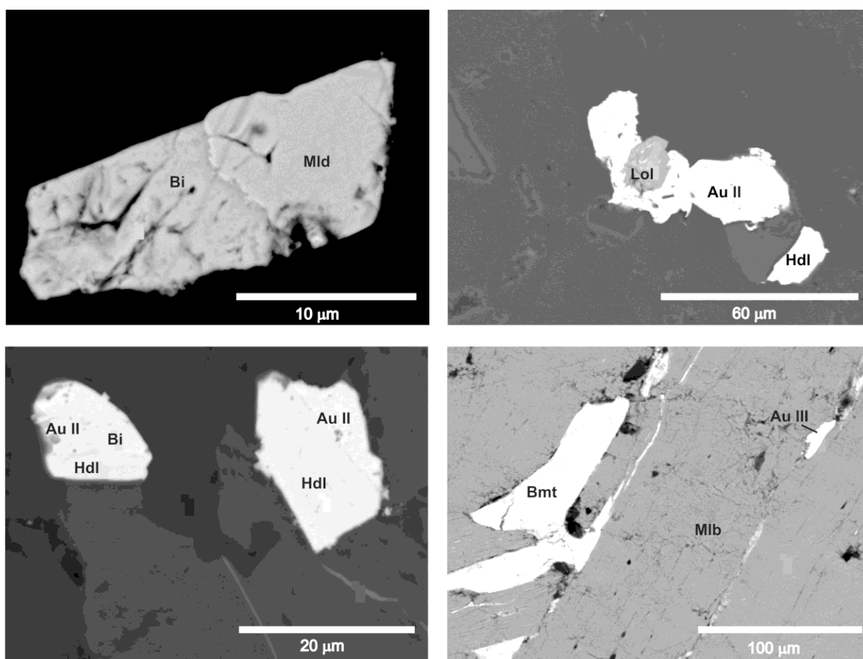
Рис. 2. Взаимоотношение минералов Мугунского рудопроявления.
