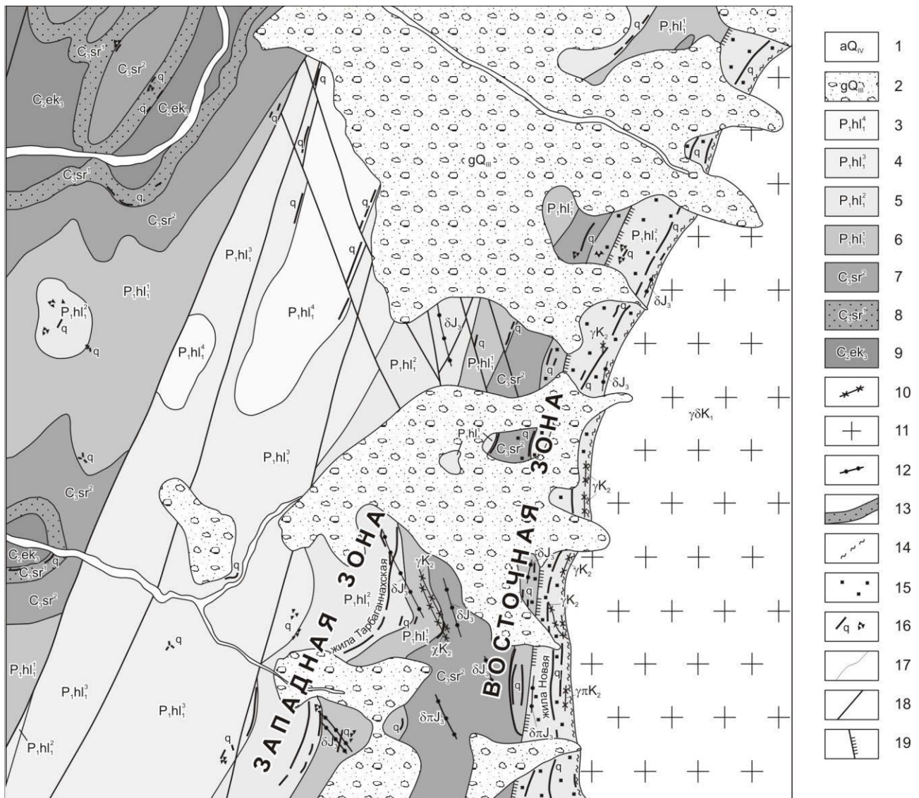
Рис. 1. Геологическая карта Мугунского рудопроявления (по Кораблеву Д.Н. и др., 1987 г., с изменениями).
